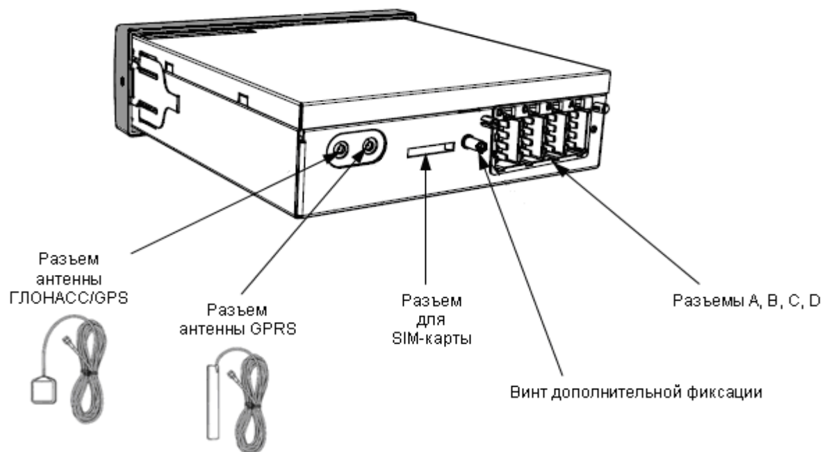
Рисунок 3 – Внешний вид задней панели КУ
