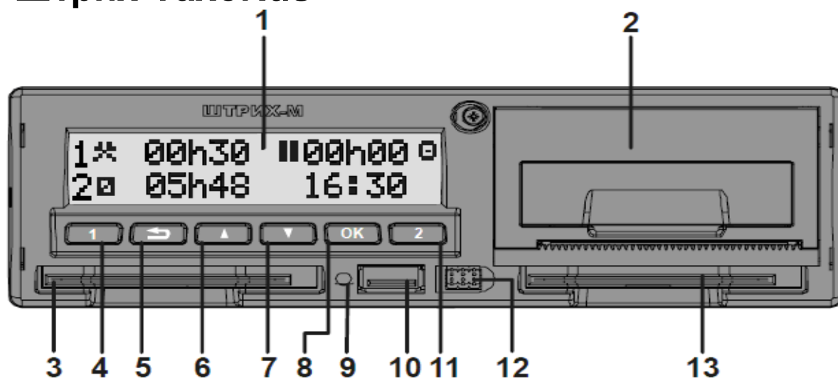
Рисунок 2 – Внешний вид передней панели КУ
